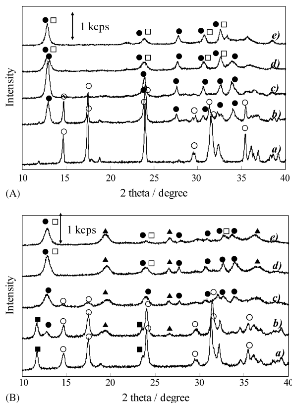
Fig. 2. XRD patterns of the precursors of the hp -Cu/Zn (A) and hp -Cu/Zn/Al (B) catalysts after the precipitation. (A) a, hp -Cu 90 /Zn 10 ; b, hp -Cu 70 /Zn 30 ; c, hp -Cu 50 /Zn 50 ; d, hp -Cu 30 /Zn 70 ; e, hp -Cu 10 /Zn 90 . (B) a, hp -Cu 80 /Zn 10 /Al 10 ; b, hp -Cu 60 /Zn 30 /Al 10 ; c, hp -Cu 45 /Zn 45 /Al 10 ; d, hp -Cu 30 /Zn 60 /Al 10 ; e, hp -Cu 10 /Zn 80 /Al 10 . (●) (Cu,Zn) 5 (CO 3 ) 2 (OH) 6 : aurichalcite; (□) Zn 5 (CO 3 ) 2 (OH) 6 : hydrozincite; (○) Cu 2 CO 3 (OH) 2 : malachite; (▲) Zn 4 CO 3 (OH) 6 ·H 2 O; (■) (Cu,Zn) 6 Al 2 (OH) 16 CO 3 ·4H 2 O: hydrotalcite.
