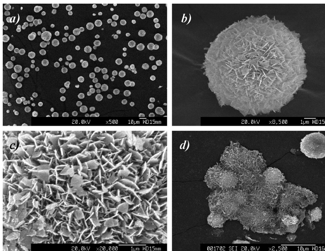
Fig. 3. SEM images of the hp -Cu 30 /Zn 70 and hp -Cu 80 /Zn 20 catalysts. Catalysts and magnifications: (a) hp -Cu 50 /Zn 50 500×; (b) hp -Cu 50 /Zn 50 8500×; (c) hp -Cu 50 /Zn 50 20,000×; (d) hp -Cu 80 /Zn 20 2500×.
